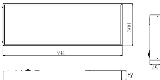
CCB-H 15 Вт IP54
